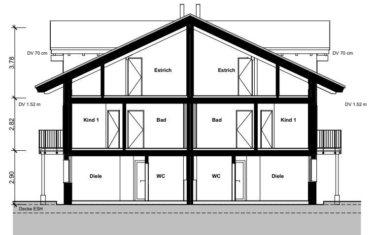
Schnitt B-B
