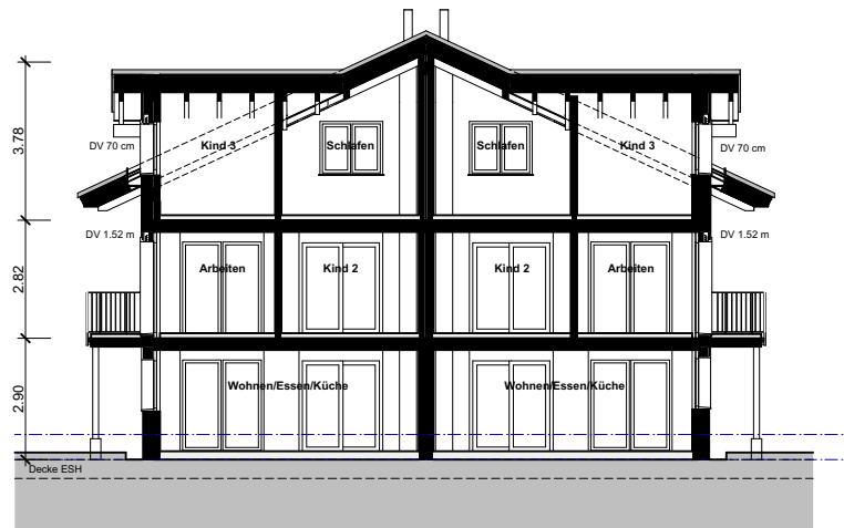
Schnitt A-A
