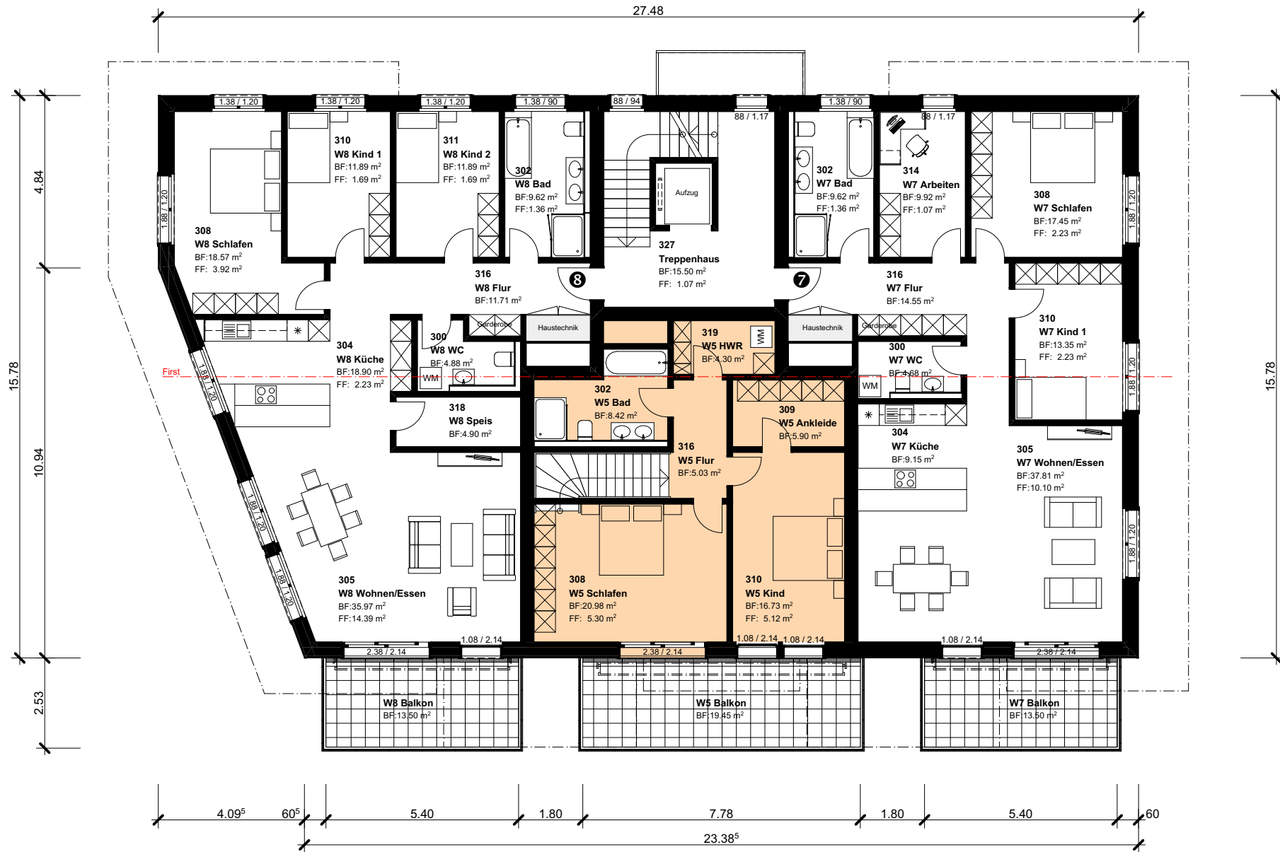
Wohnung 8 Bruttofläche 156.16 m 2
