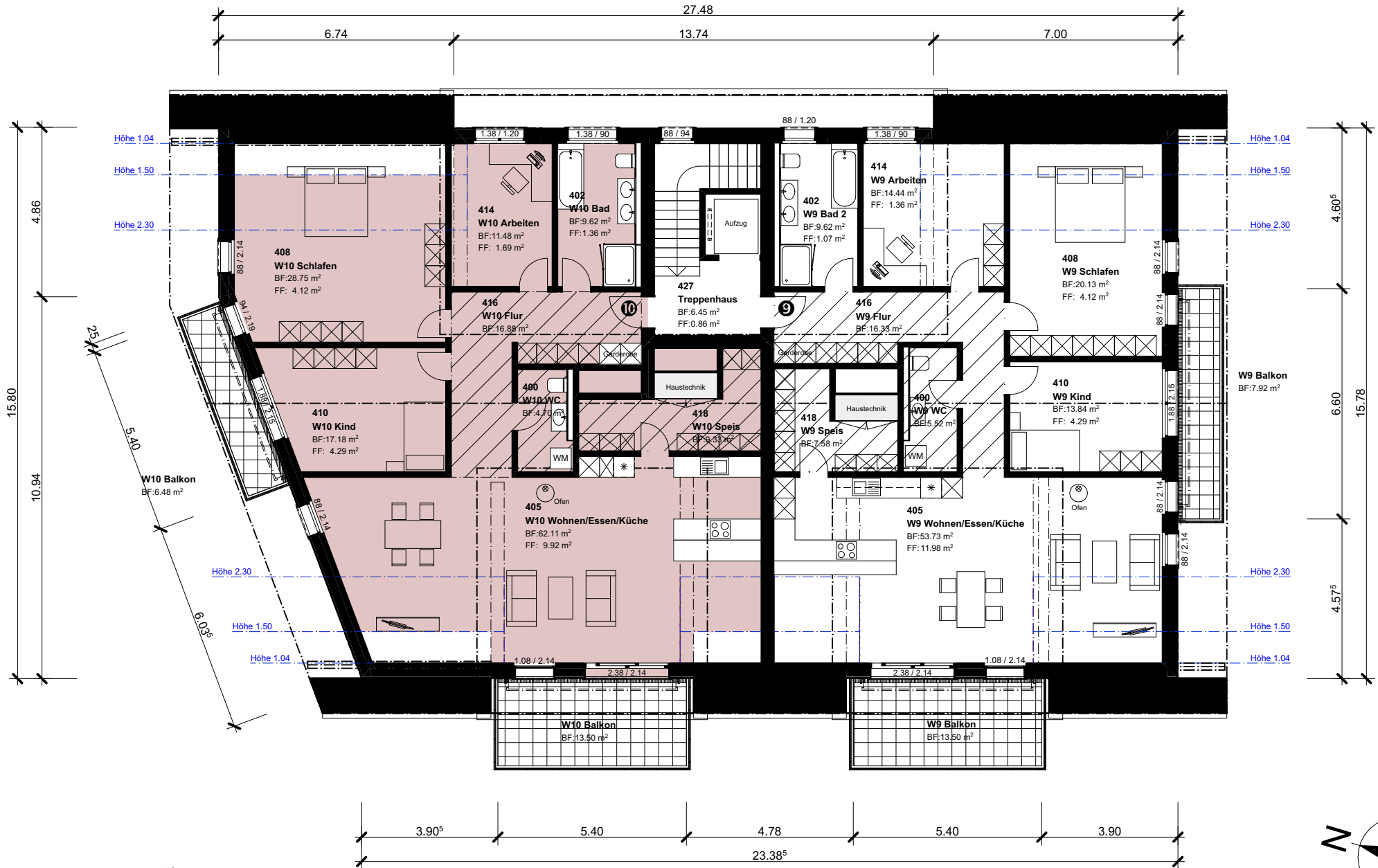
Wohnung 10 Bruttofläche 187.44 m 2
